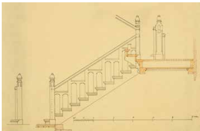
Tegninger fra det begrænsede tegningsmateriale, der er fundet. Til venstre ses detalje fra hovedhusets trappe. Til højre et udsnit af tinghuset facade.
